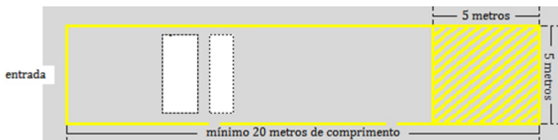
Figura 3 - Pista de Ensaio com Simulador de Pista
